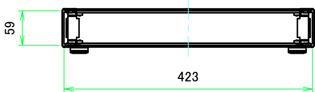
B-B ( 1:6.5 )
