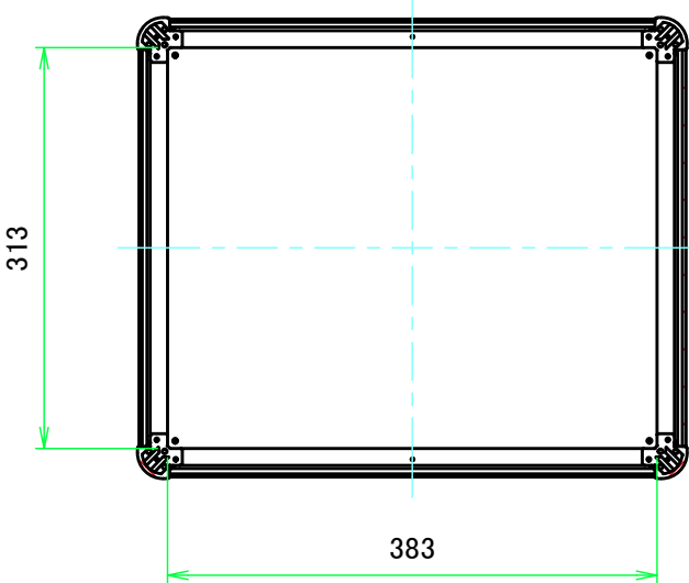
C-C ( 1:6.5 )
